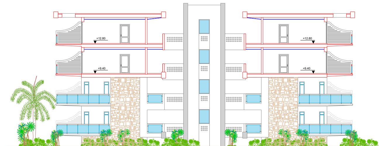
SECCION 2 (bloque 1)
