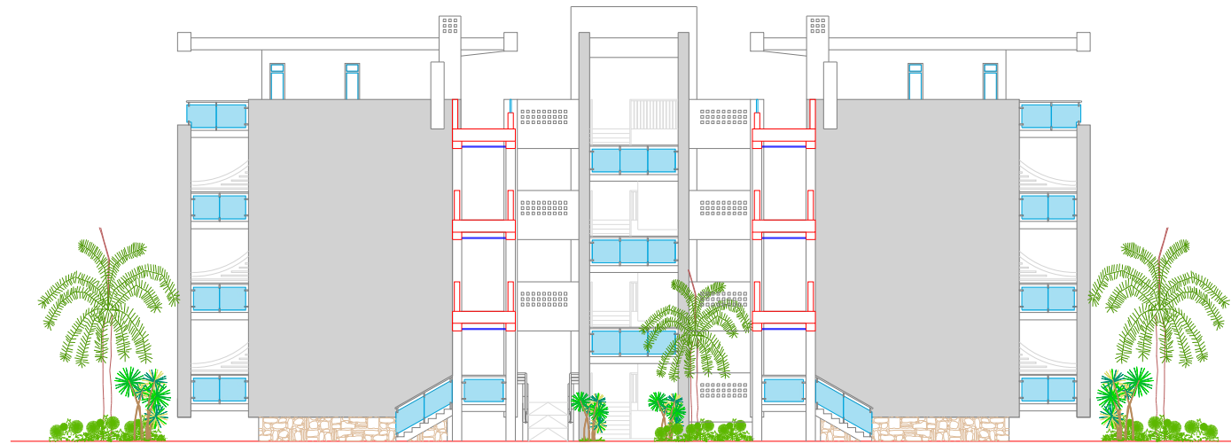
ALZADO 3 (bloque 1)
