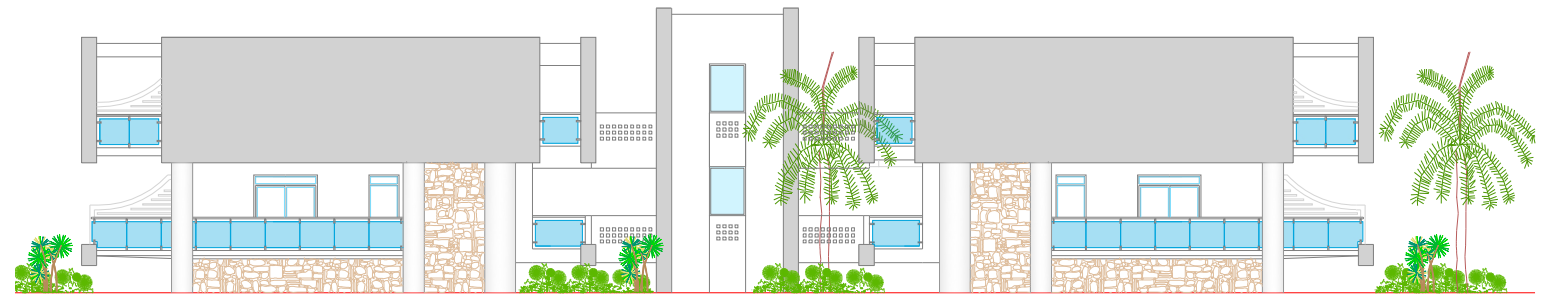
ALZADO 3
