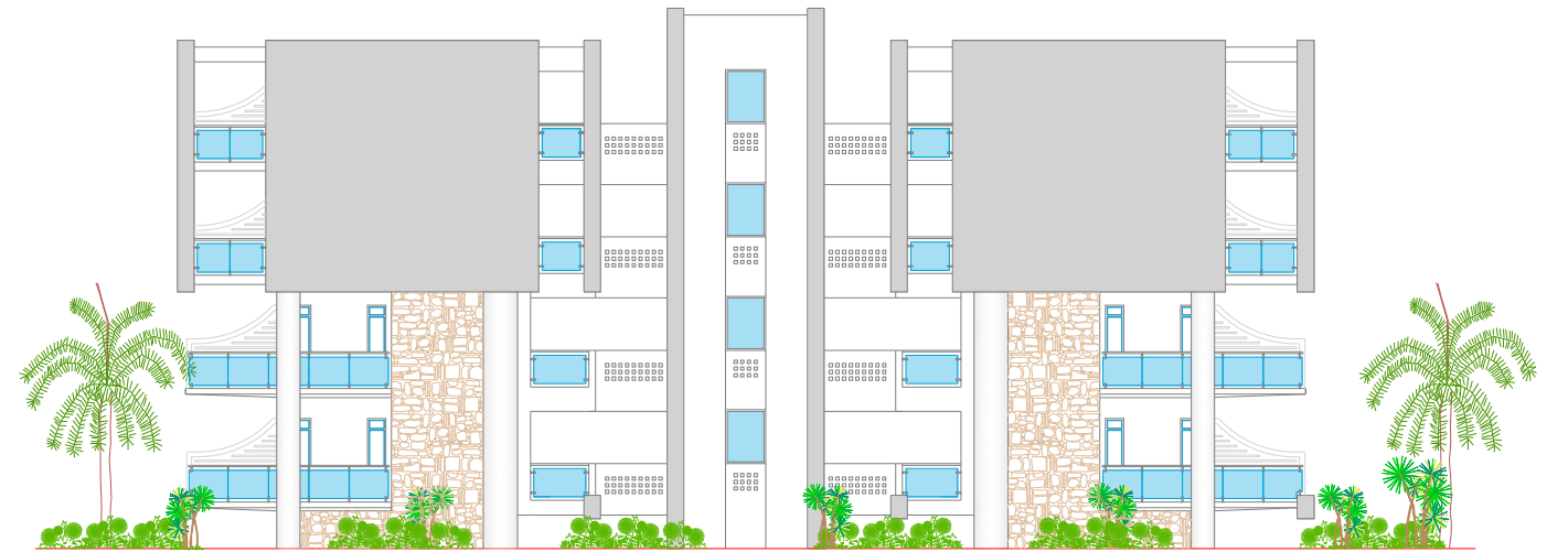
ALZADO 4 (bloque 1)
