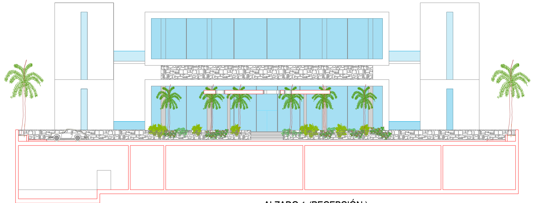
ALZADO 1 (RECEPCIÓN)
