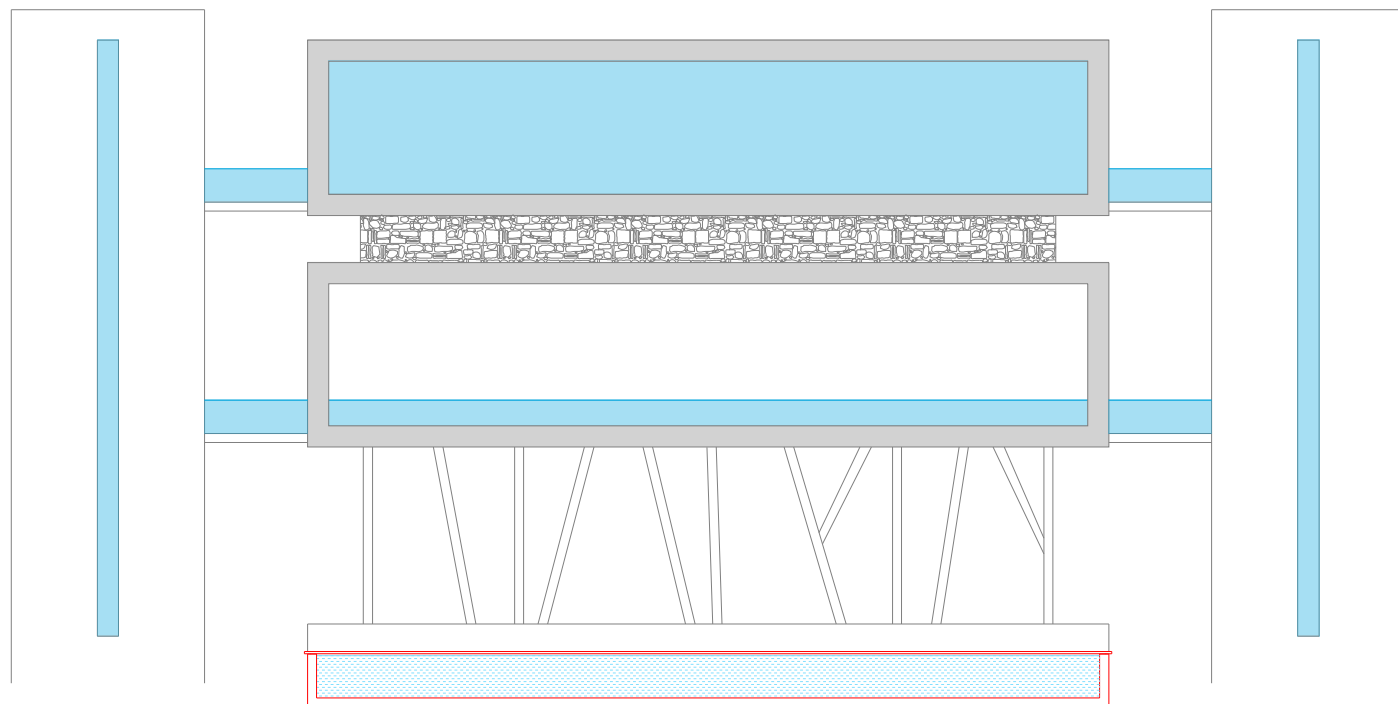
ALZADO 2 (RECEPCIÓN)
