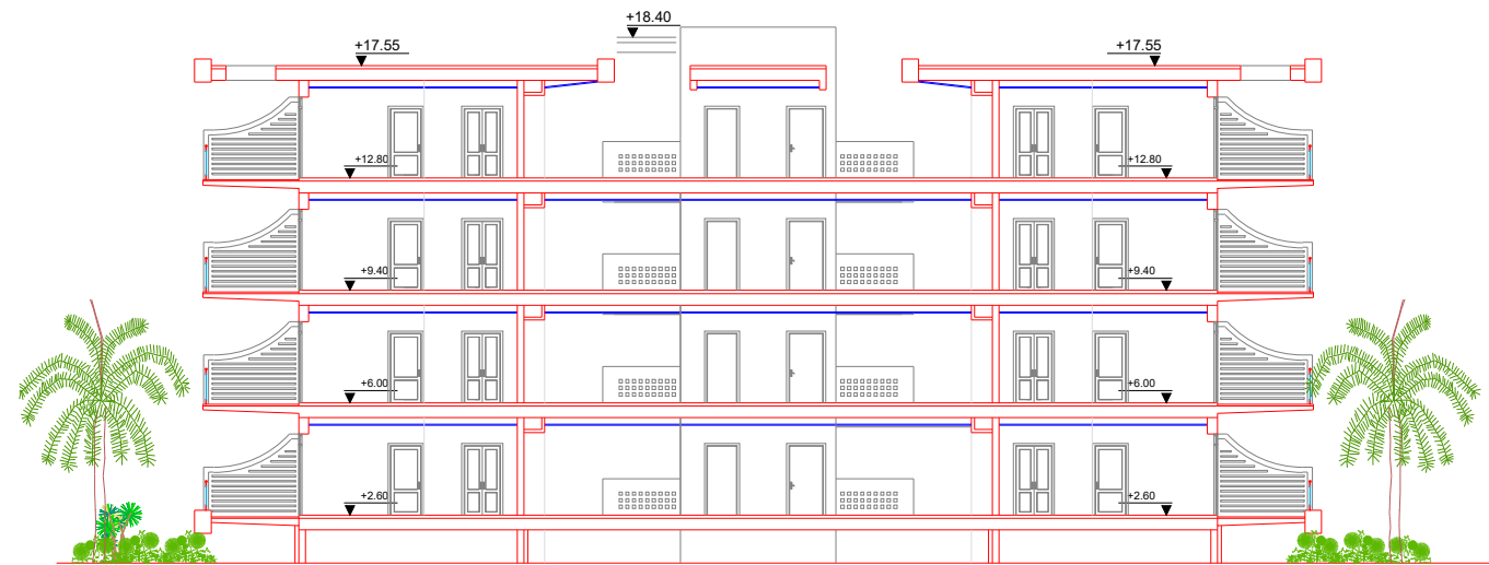
SECCION 1 (bloque 1)
