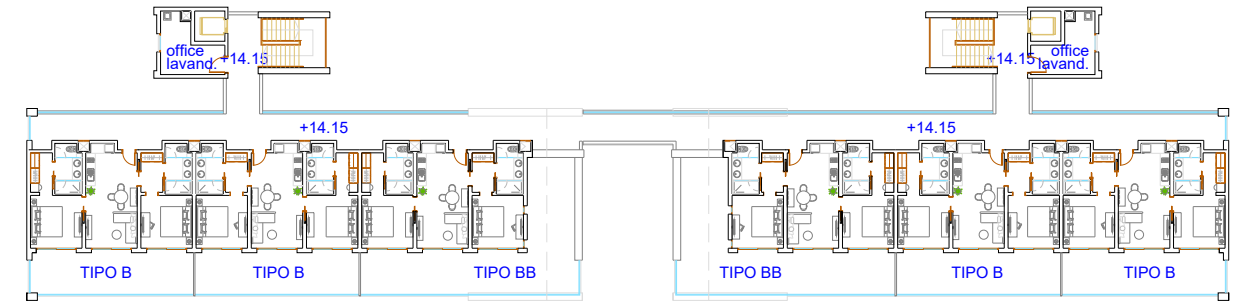
NIVEL 4
