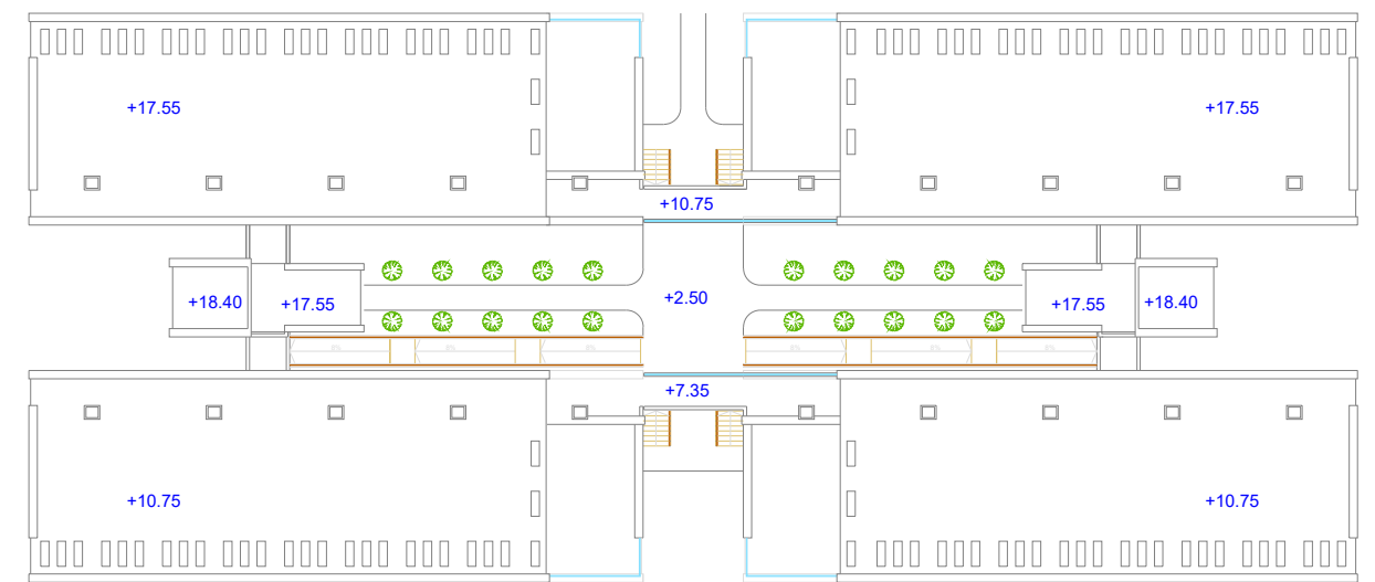
CUBIERTA GENERAL
