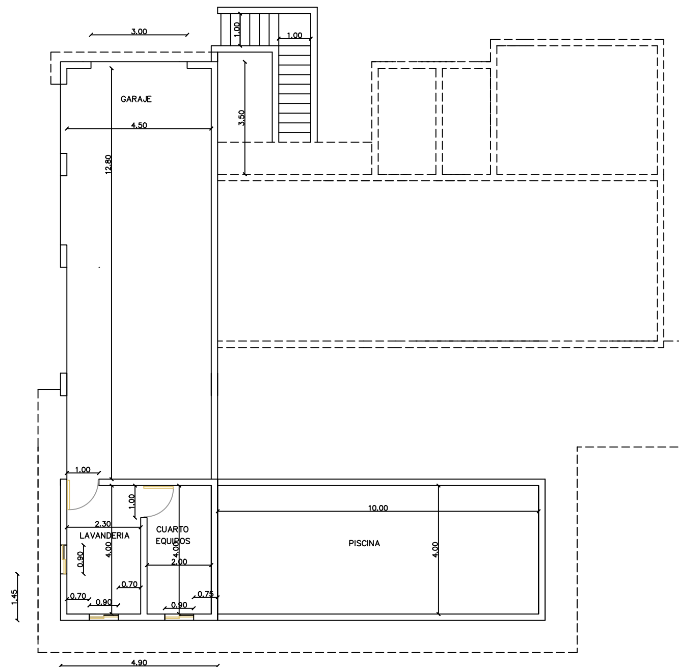
1 PLANTA DIMENSIONADA NIVEL INFERIOR A-5
