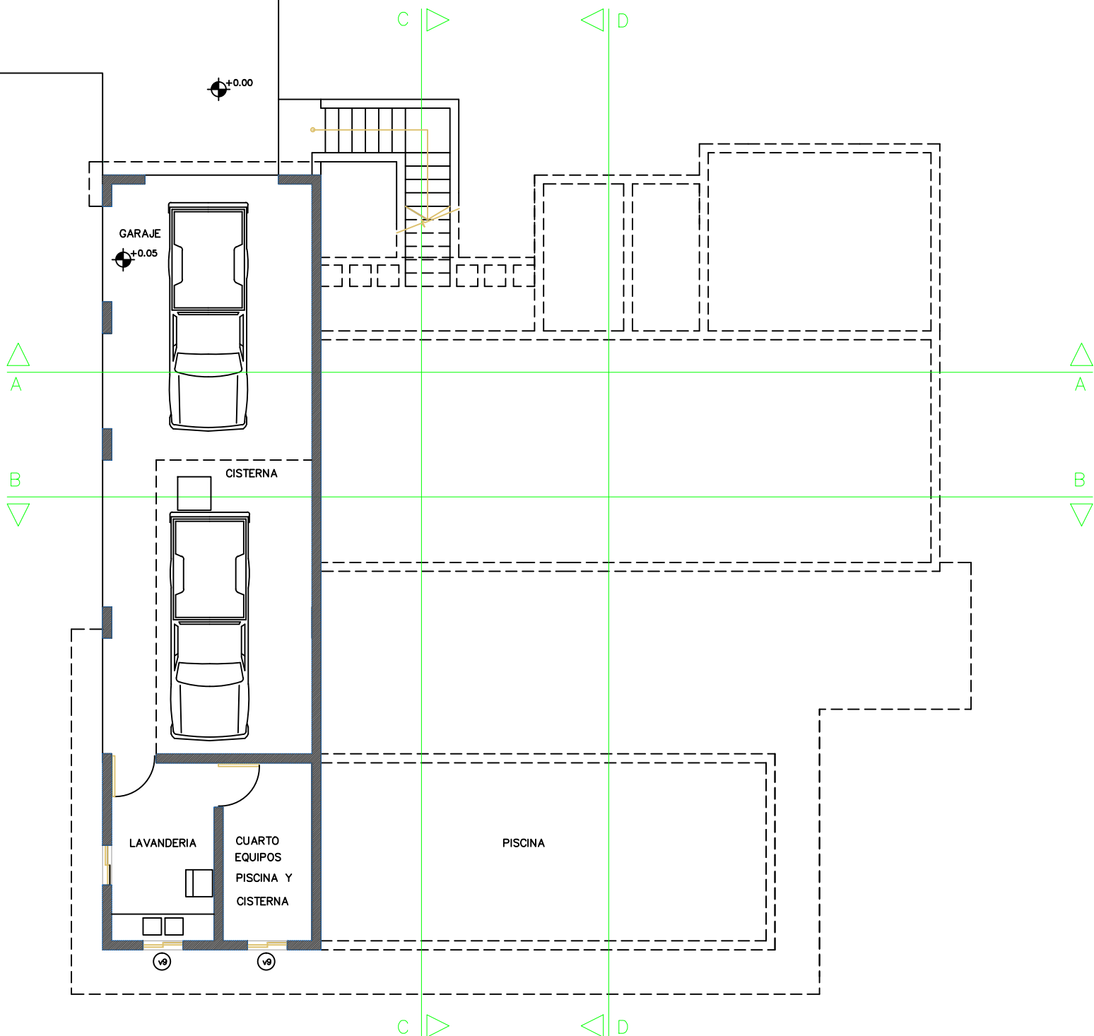
1 PLANTA ARQUITECTONICA NIVEL INFERIOR A-2 ESCALA GRAFICA 1mt 2mt 4mt
