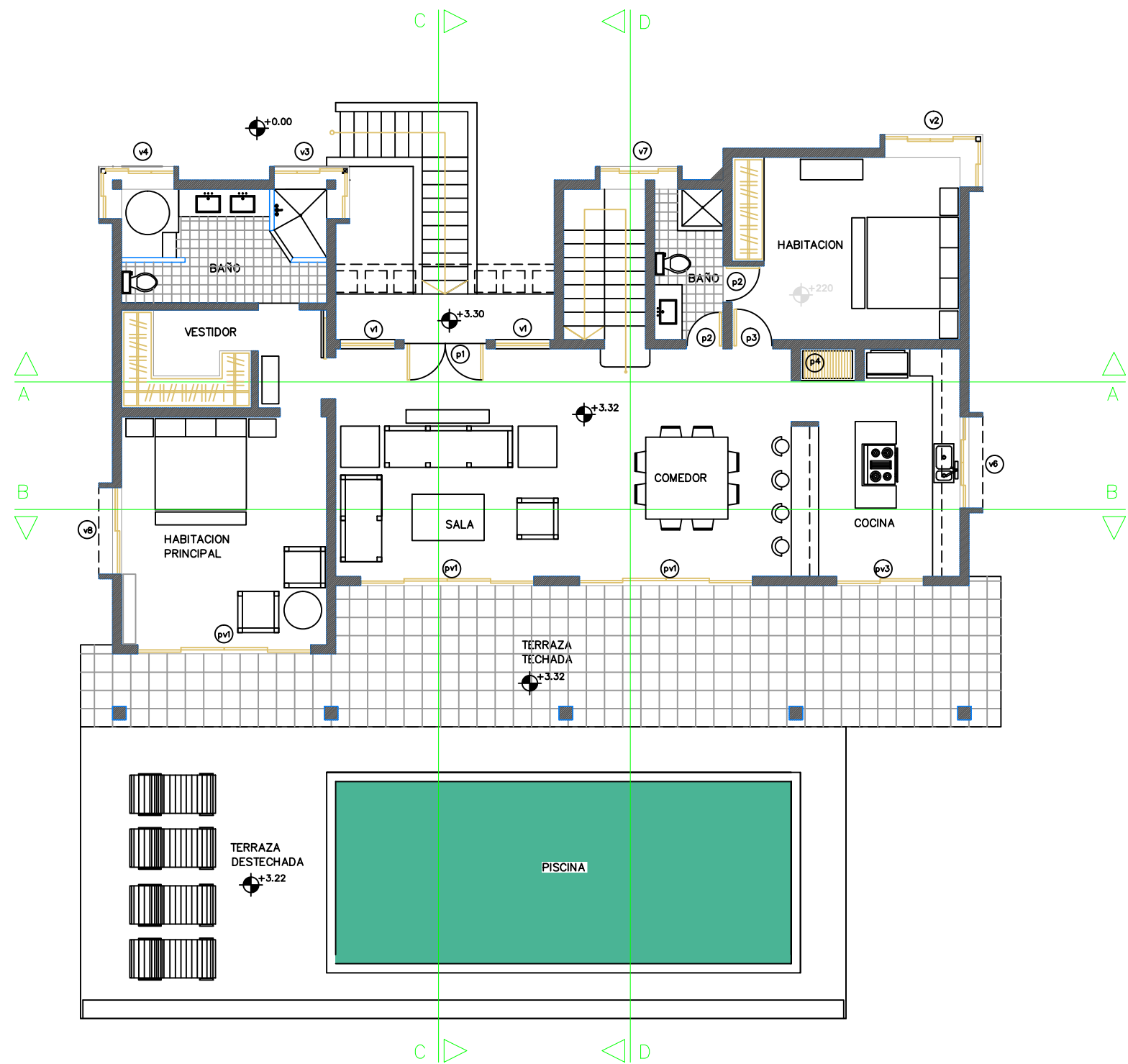
1 PLANTA ARQUITECTONICA NIVEL INGRESO A-3 1m 2m 4m ESCALA GRAFICA
