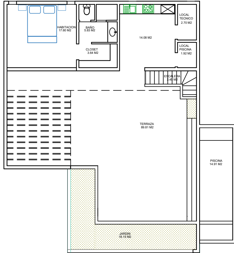
PLANTA ARQ. NIVEL 02 TECHO TERRAZA C1
