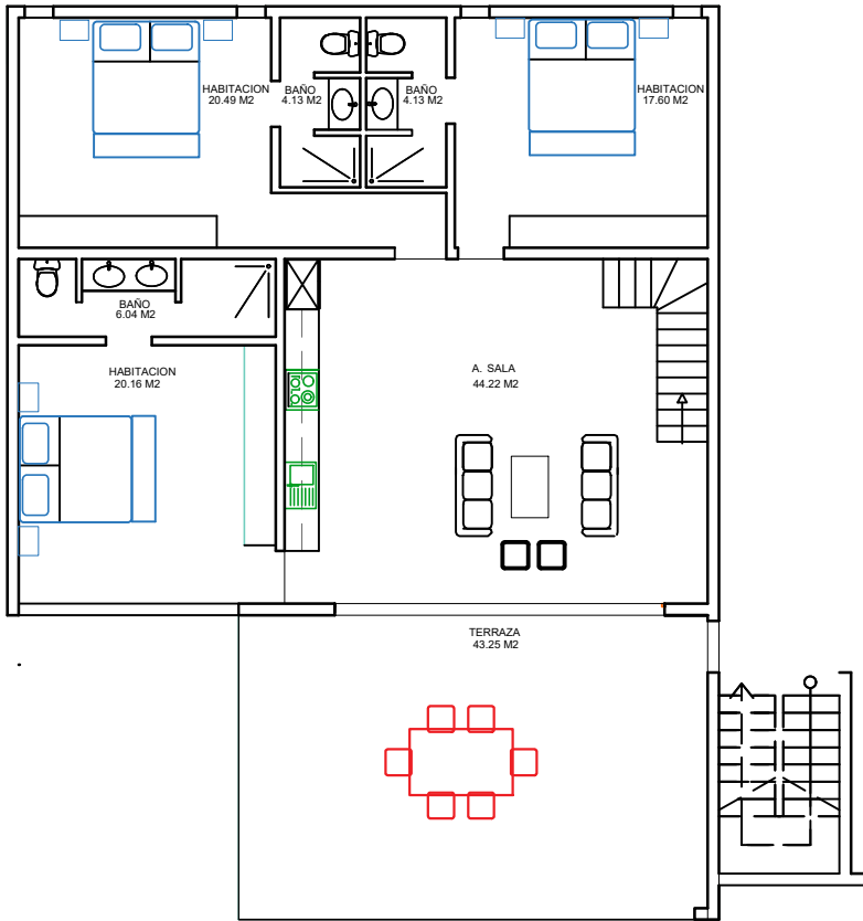
PLANTA ARQ. NIVEL 02 C1
