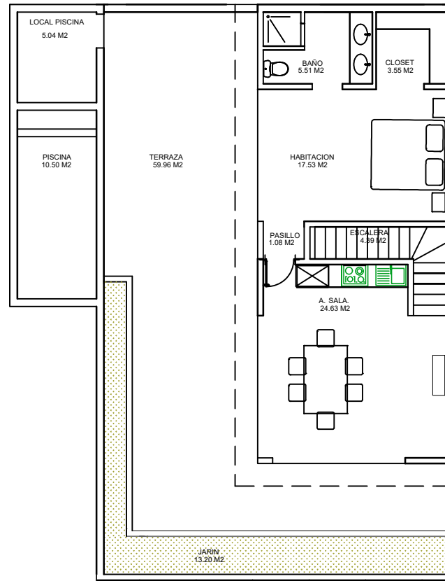
PLANTA ARQ. NIVEL 02 TECHO TERRZA C2
