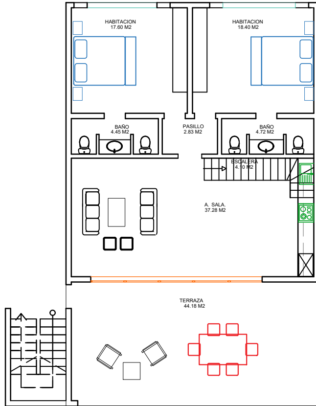
PLANTA ARQ. NIVEL 02 C2
